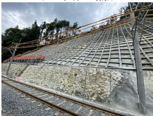
運転再開に必要な施設の復旧完了の状況 (2021年8月26日撮影)
